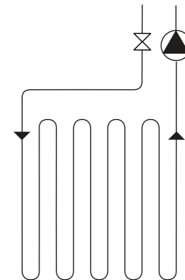
Fig 3: Principdiagram for tilslutning direkte på varmesystemet via ventil med forindstilling. (Kun små baderum)
