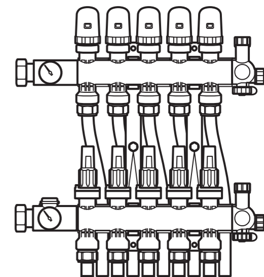
Fig 4: Traditionel tilslutning via Uponor fordelerrør 3/4" eurokonus. Regulering sker med telestater og kontrolenhed med rumtermostater.
