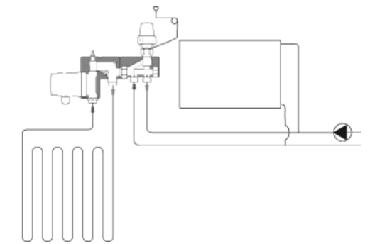
Fig 2: Principdiagram for 2-strengs anlæg med Uponor Fluvia Push 12.
